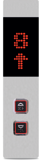
PX 170 DM Kapak (Cover) : 90*390 mm Kutu Box: 70*310
